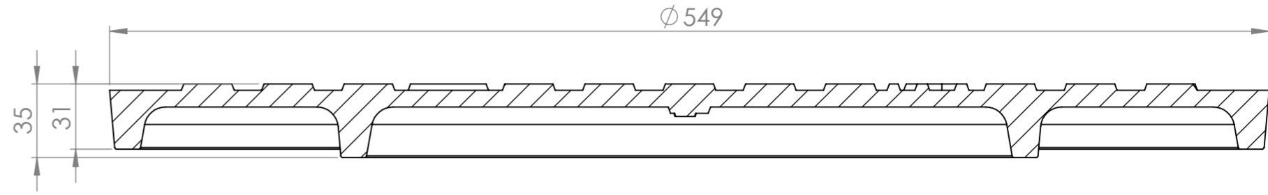
SECTION A-A
