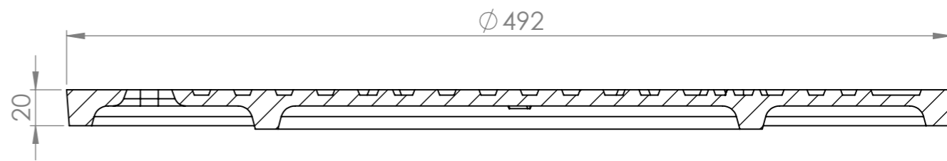
SECTION A-A SCALE 1 : 3
