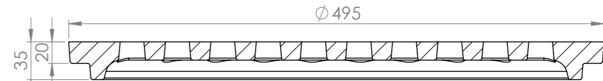
SECTION A-A
